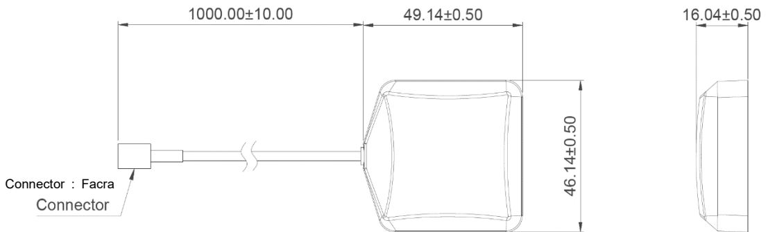
図2.5-7 GNSS Antenna
