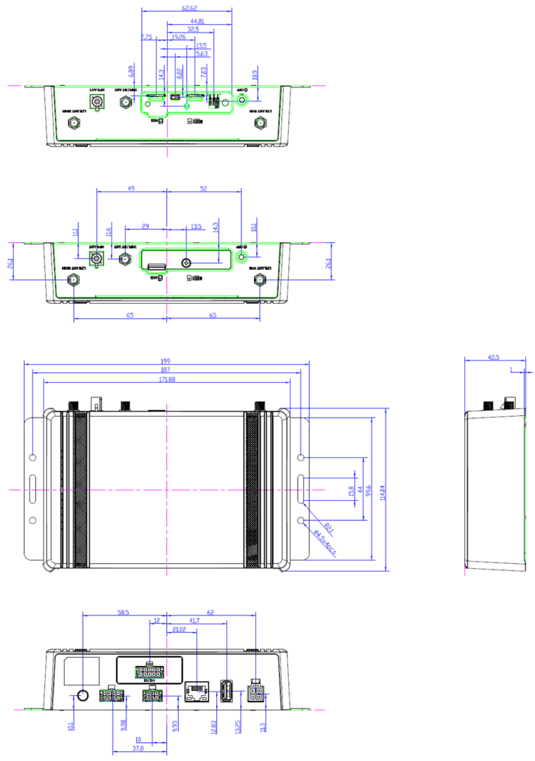
図2.1-1 筐体寸法図
