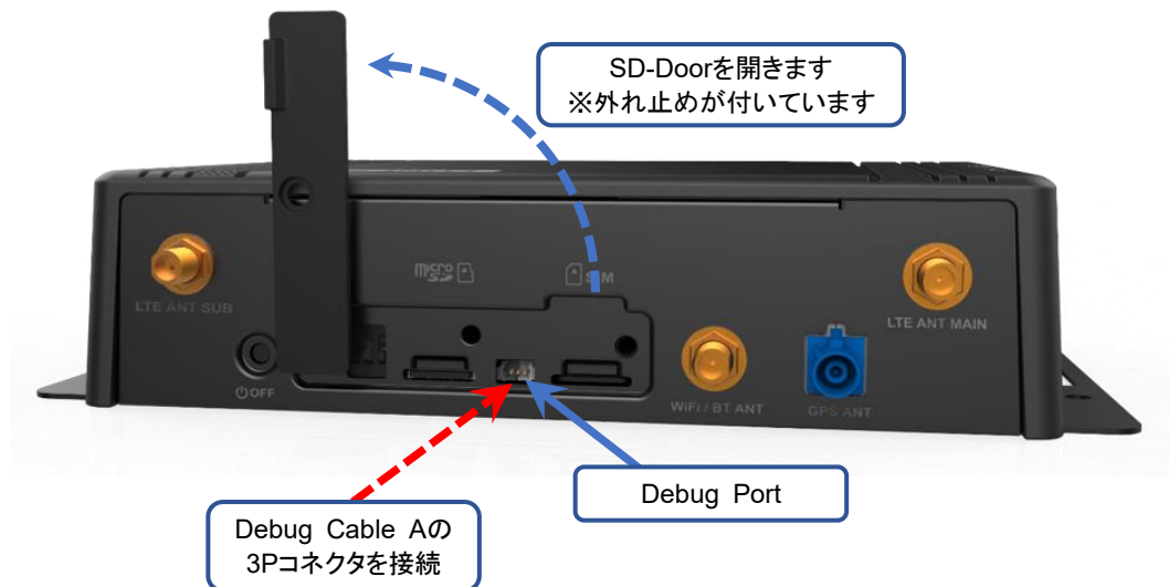
図7.2-1 本体へのDebug Cable接続
