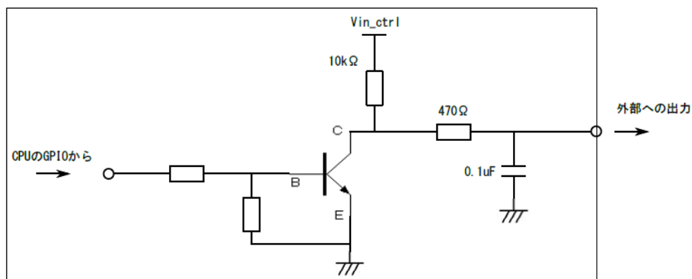
図4.7-2 DO回路図
