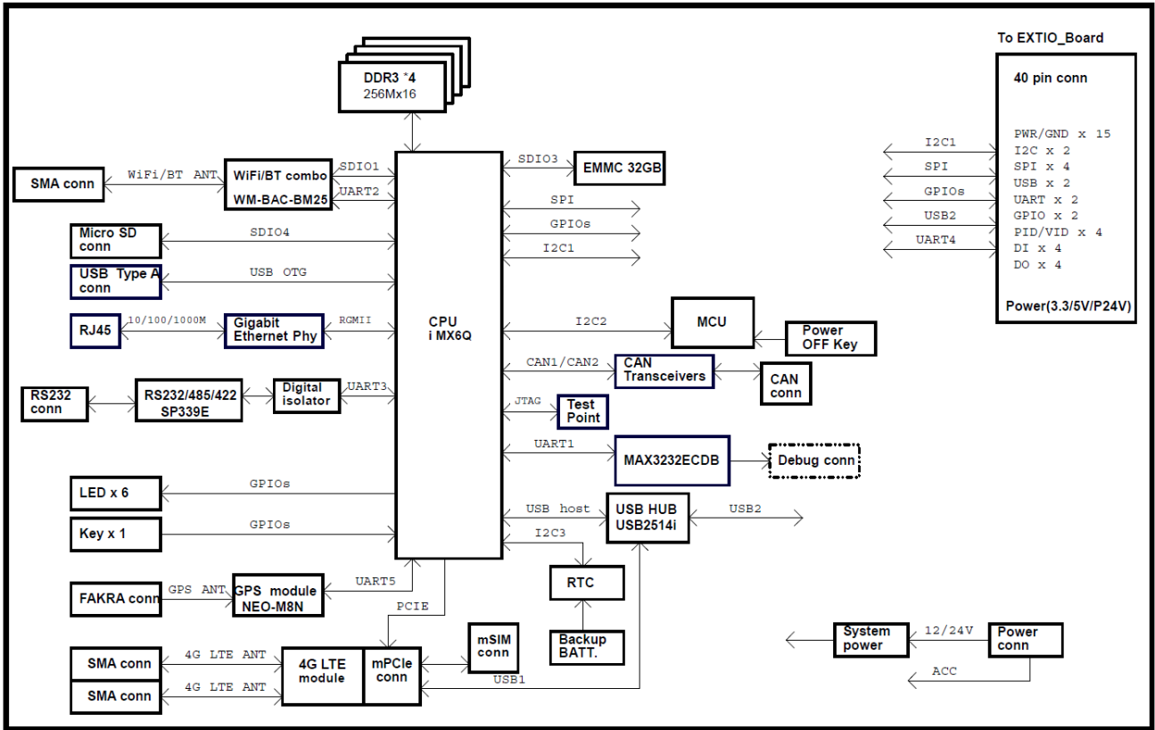
図2.3-1 ブロック図
